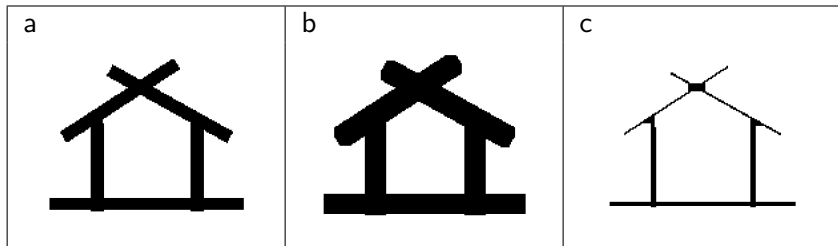
Figura: Exemplo das operações morfológicas básicas: a) a imagem binária original, b) o resultado da dilatação por uma círculo digital de raio 3, e c) o resultado da erosão pelo mesmo círculo digital.
